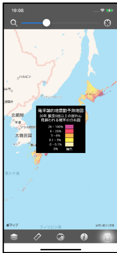
確率論的地震動 予測地図
