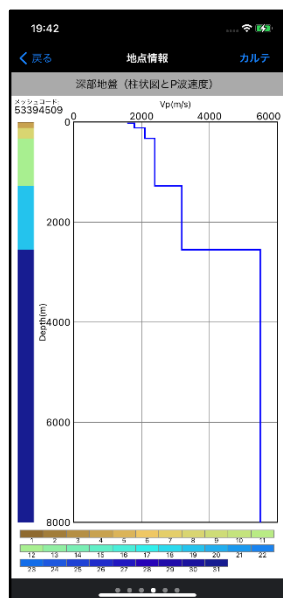
深部地盤 (P波速度)
