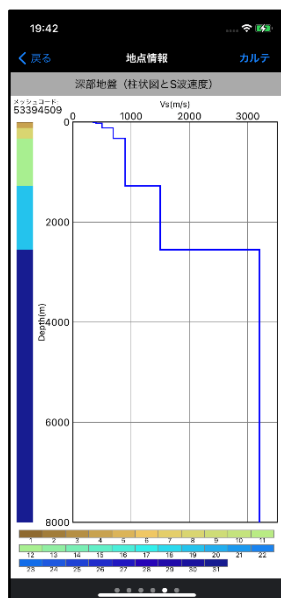
深部地盤 (S波速度)
