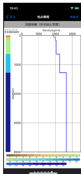
深部地盤 (密度)
