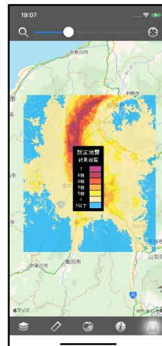
想定地震地図
