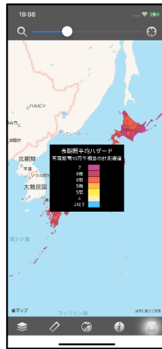
長期間平均 ハザード地図
